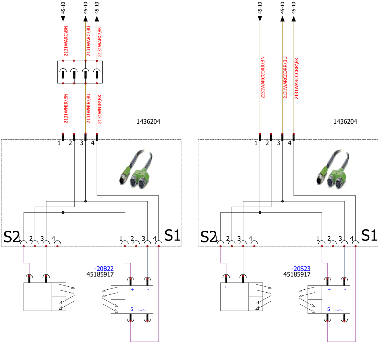
ARC LAMP JAM SENSOR CROSS SENSOR DE ATASCO DEL ARC LAMP CRUZADO
