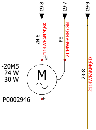
Belt Motor Fan Up Ventilador superior del motor de la banda
