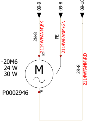
Belt Motor Fan Down Ventilador inferior del motor de la banda
