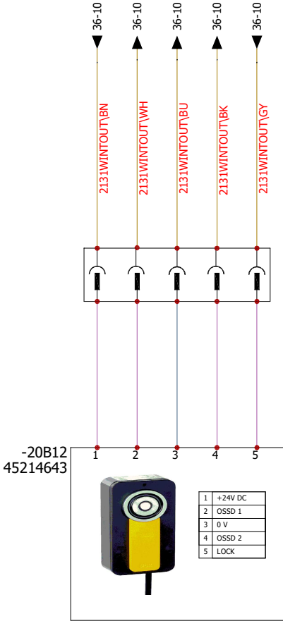
Safety Interlock Front OUT Bloqueador de seguridad frontal de salida
