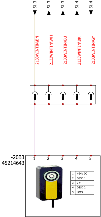
SAFETY INTERLOCK BACK 1 BLOQUEADOR MAGNETICO TRASERO 1
