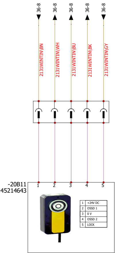
Safety Interlock Front IN Bloqueador de seguridad frontal de entrada
